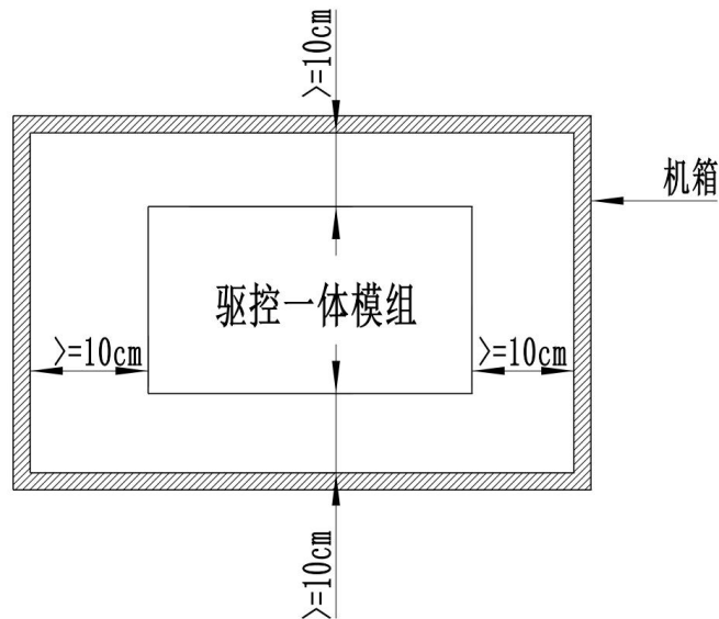
*安装空间要求图示*
