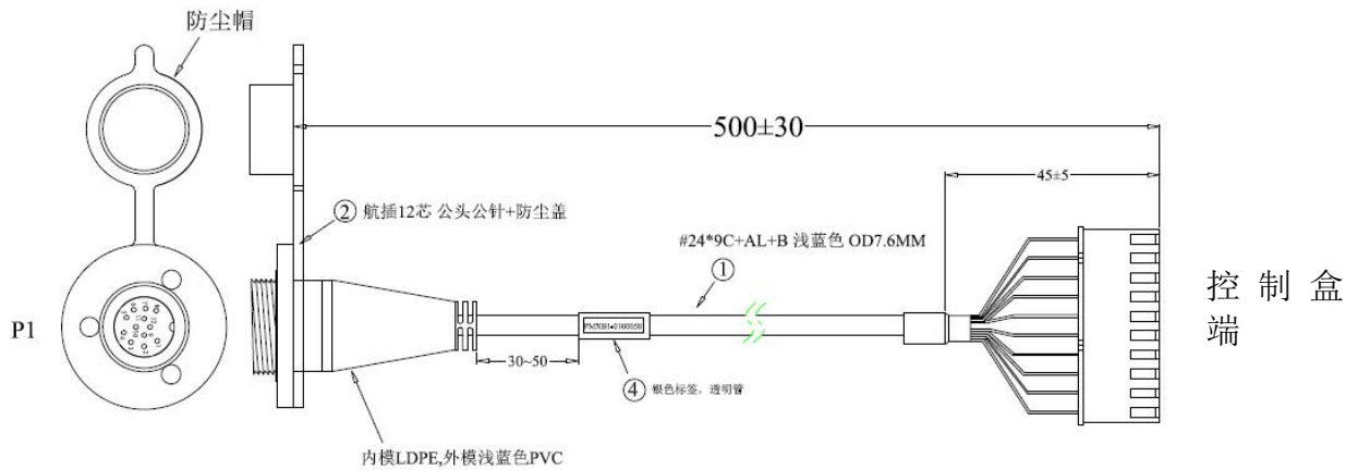
品名: 12P航空头转接线 L=0.5M
